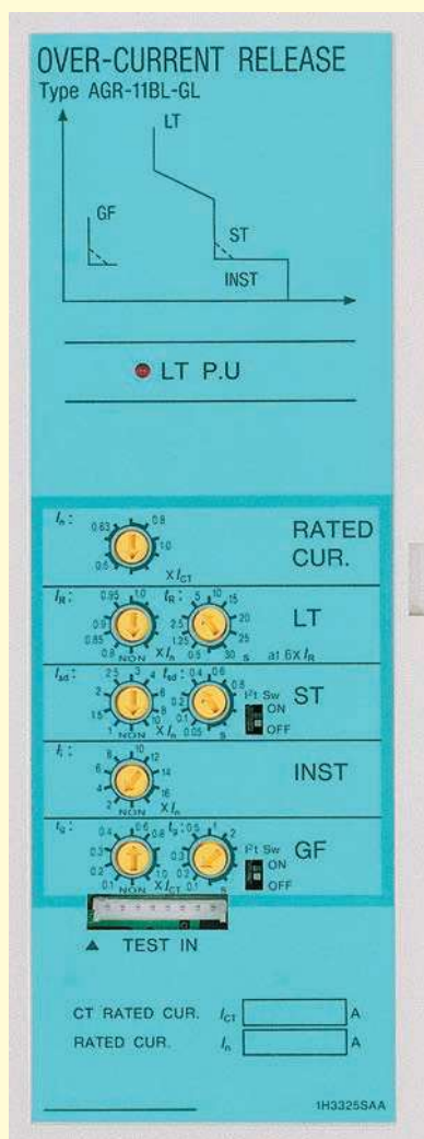
Relé estándar con ajuste por dial. Tipo AGR-11B.
