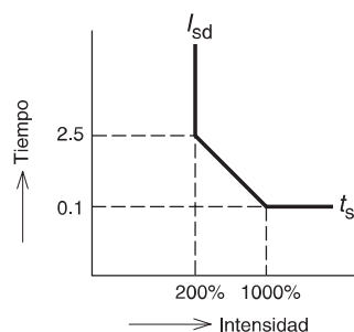
Curva característica de rampa (característica L ó R)
