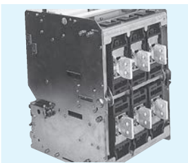
▲ Terminales verticales
