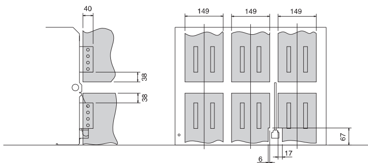
Vista posterior
