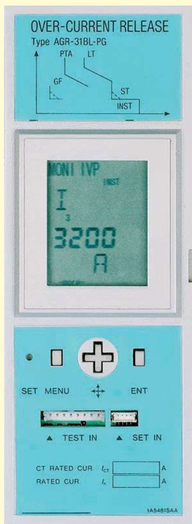
Relé especial con pantalla LCD iluminada-Analizador de potencia Tipo AGR-31B.
