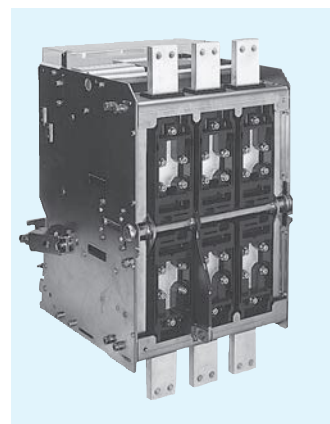
▲ Terminales frontales
