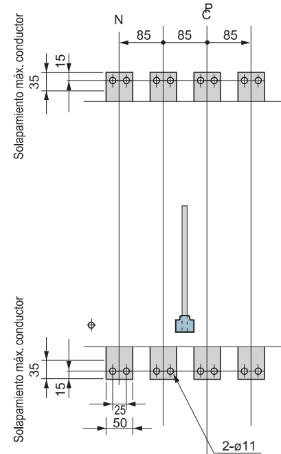
Conexión Frontal
