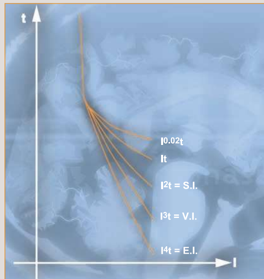
Curvas de tiempo inversa definida (I.D.M.T.) "Inverse definite minimum time"
