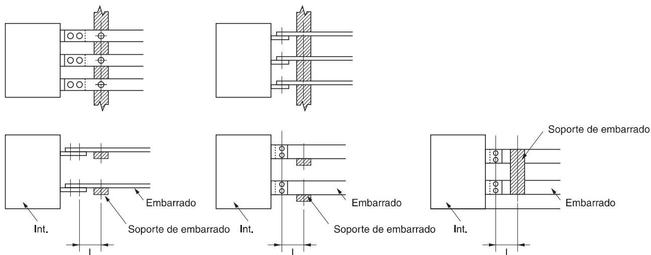
Terminales horizontales
